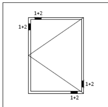
Sidohängt
