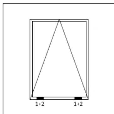
Underkantshängt fönster
